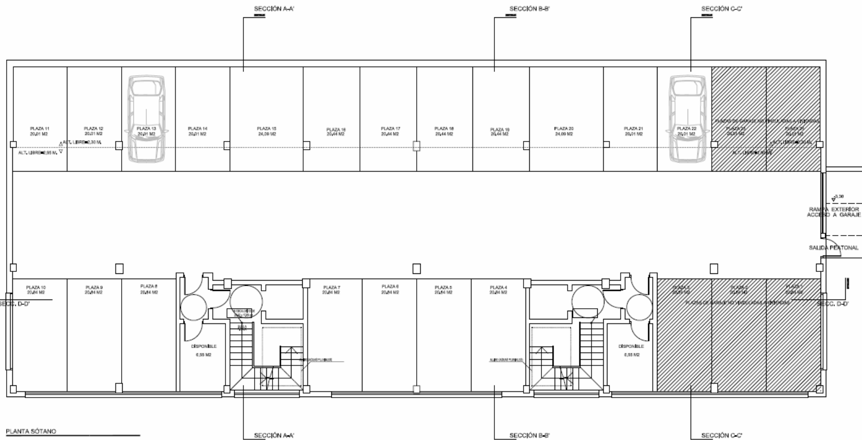
PLANTA SÓTANO
